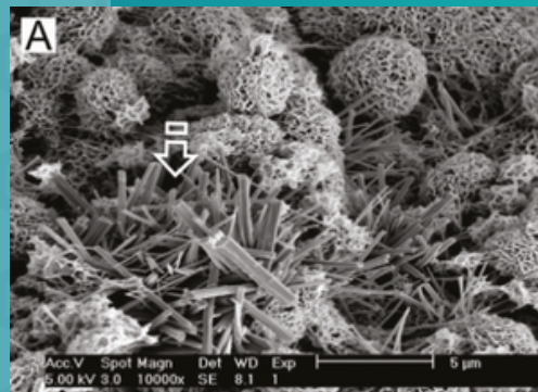
Cristaux précipités de phosphate de calcium dispersés à la surface du ciment de silicate tricalcique hydraté 1 .
